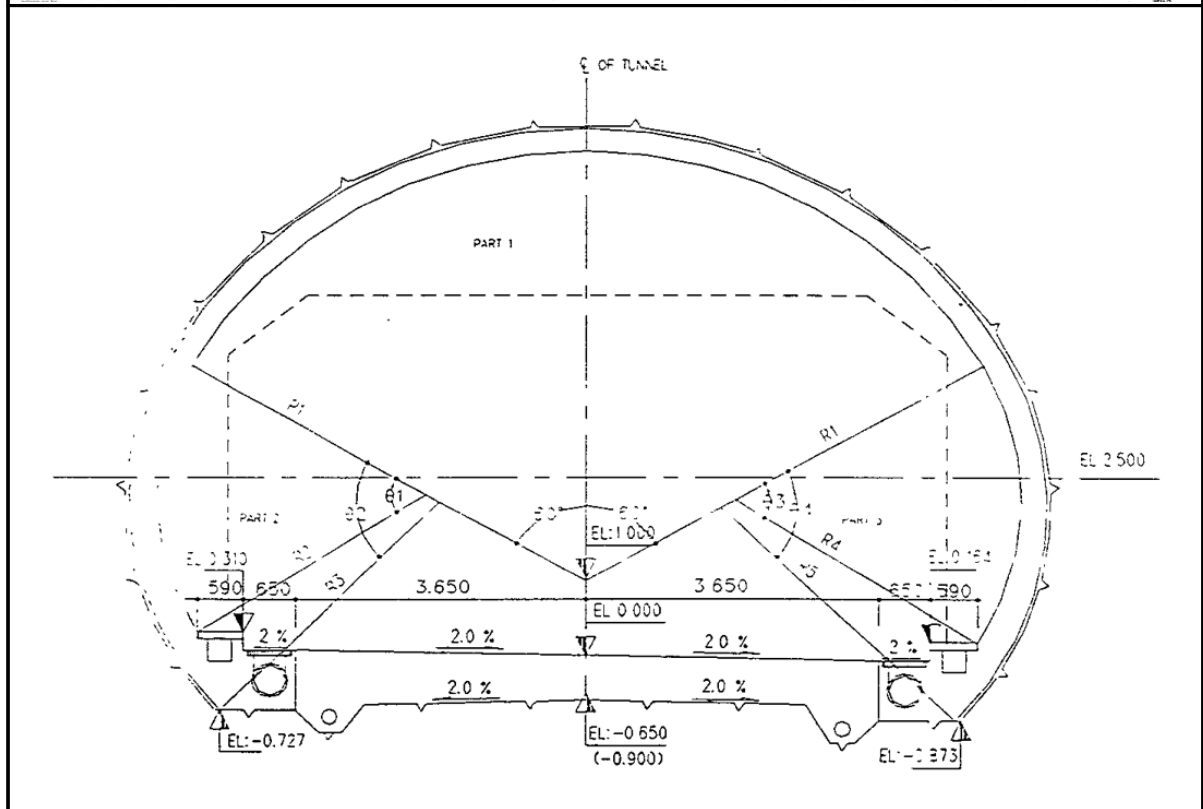
【그림】 터널 단면도
